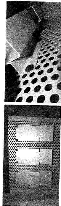
Obr. 1.3 – klobouk stojanu s prvky pro uchycení (např. samořeznými šrouby; přichycení pouze pomocí plastových špičtek není přípustné)
