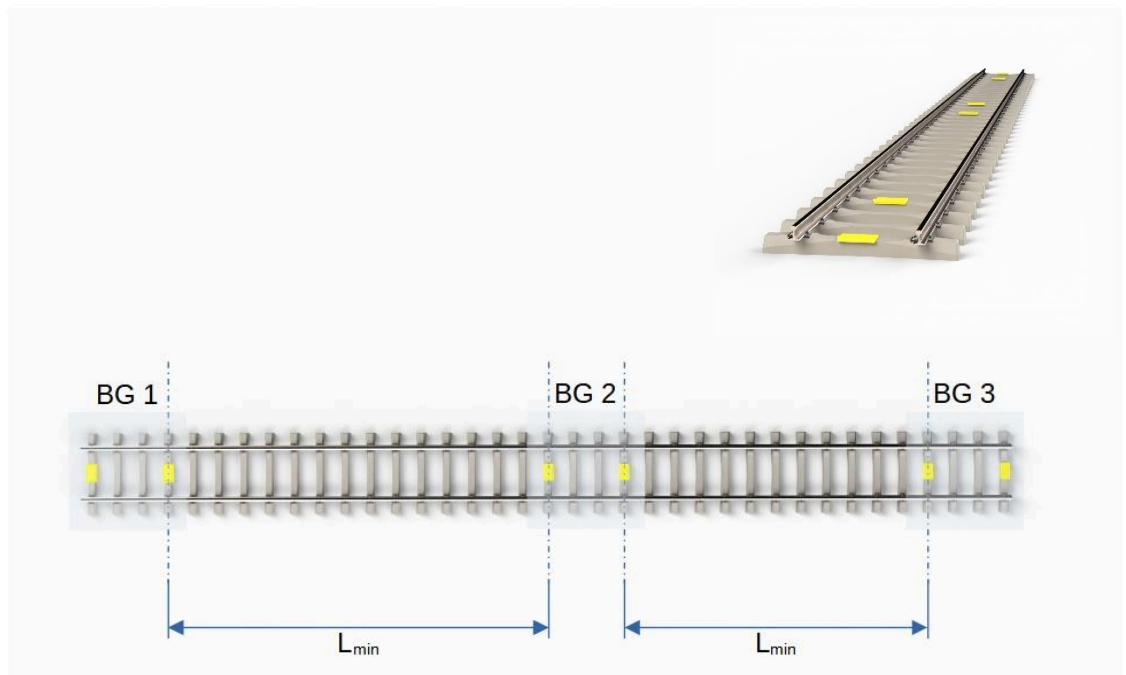
Obrázek 2 Vzdálenost balízových skupin
