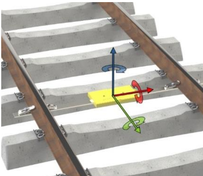
Obrázek 4 Osy
