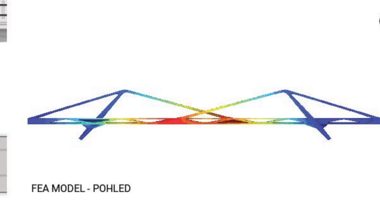
FEA MODEL - AXONOMETRIE
